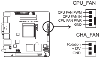
M4A88T-I DELUXE fan connectors
